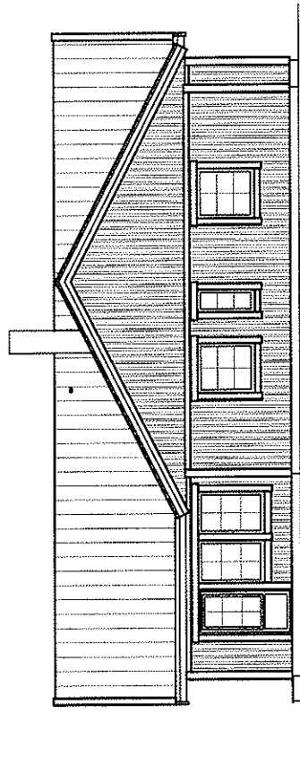
FASAD 3
